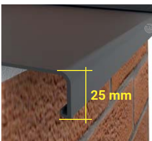
FBS 25 = Tropfkante vorne 25 mm
